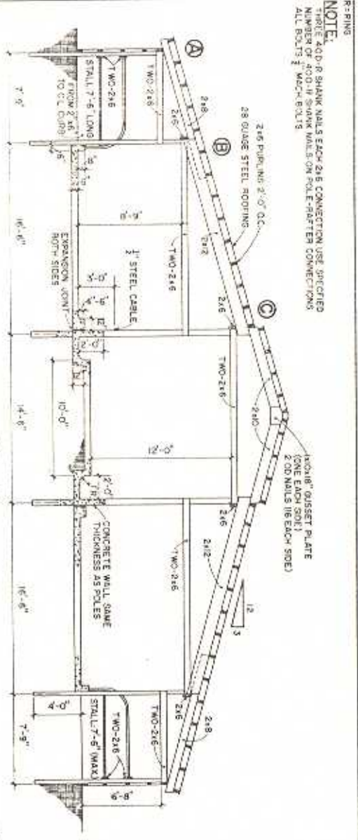
SECTION "A-A" SCALE: 1" = 4'-0"
