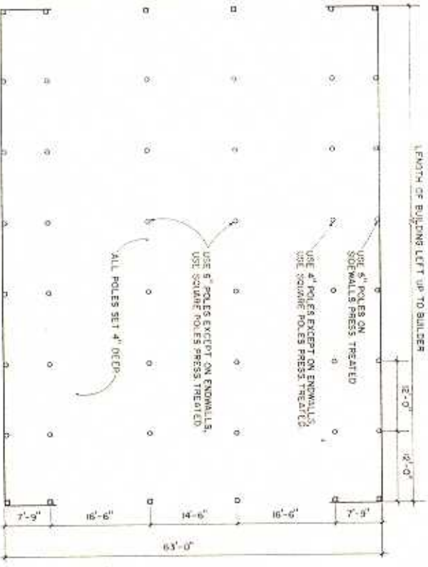
FLOOR PLAN SCALE: 1" = 12'-0"
