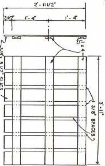
EDGE VIEW
