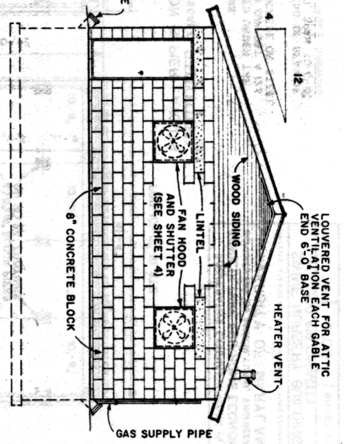
END ELEVATION
